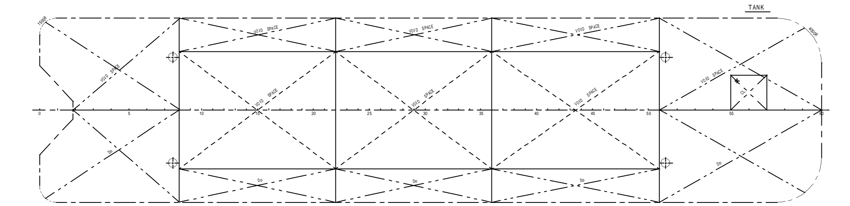
2700M 3 BOX BARGE 一般配置図
